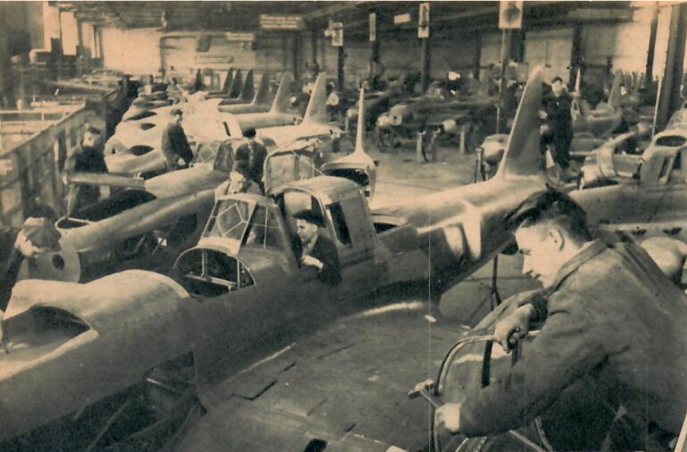
T. v.: Interiör från en rysk flygplansfabrik. För tillfället är det Iljushin-2 som är föremål för serietillverkning. Lägg märke till porträtten av Rysslands store på pelarna runt om i lokalen. — Nedan: Ett par kvinnliga radiotelegrafister tar flyg till sin arbetsplats, staden Amderma i nordligaste Ryssland.
