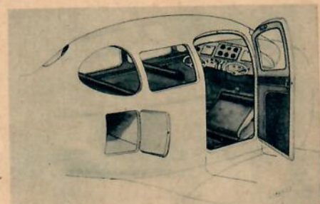
Bortsett från det infällbara landstället är den fyrsitsiga Ercoupe ganska lik sin välkända föregångare.
