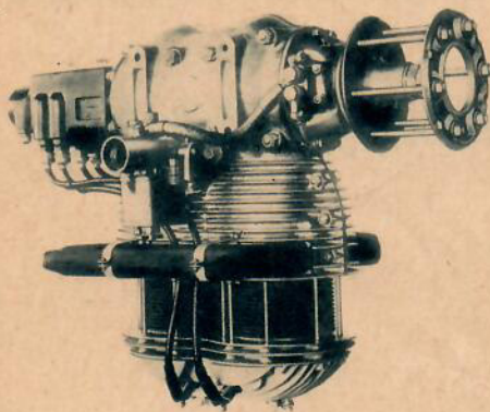
Walter A heter en ny hjälpmotor för segelflygplan på 22 hk. Motorn existerar tyvärr ännu så länge endast i prototyp, men serie-tillverkning lär vara under uppläggning.
