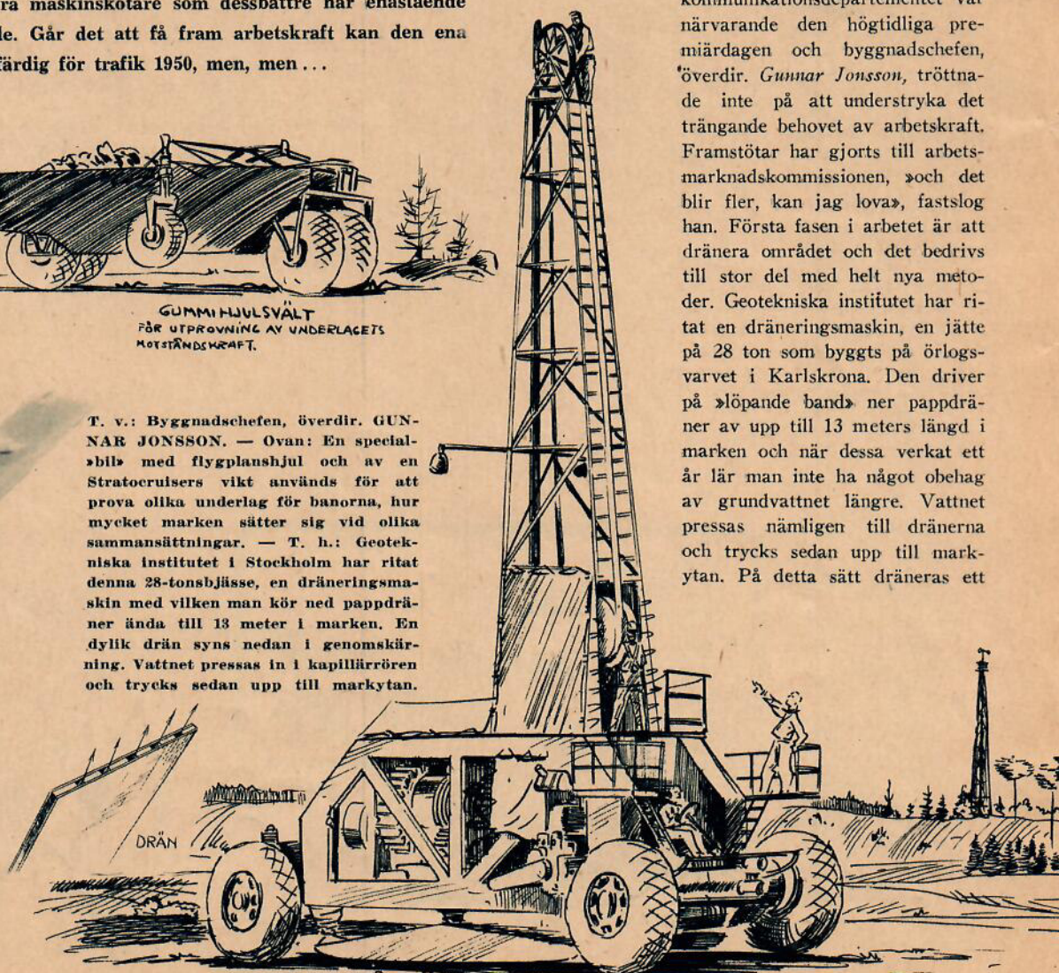
DJUPDRÄNERINGSMASKIN STÖRRE MODELLEN (MED 13-METERSTORNET)
