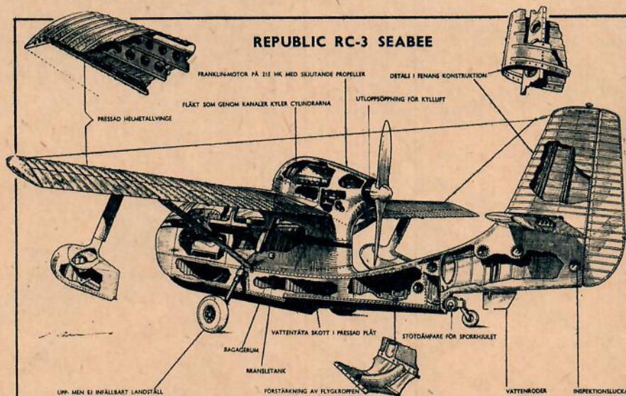
Ovan en röntgenteckning av Seabee. Propellern på teckningen är som synes av den gamla fasta typen. Serierversionen har emellertid en reversibel Hartzell-propeller. — Nedan en bild från demonstrationen av Seabee på Bromma.
