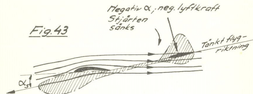
Om flygplanet skulle flyga i stabilisatorns O-riktning, skulle nedsvepningen bakom vingen sänka stjärten.
