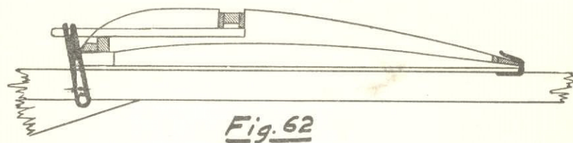
Enkel och effektiv vingfastsättning. Bakkanten hålls i läge av en bygel av t. ex. en hårnål. Främre delen kan byggas in för att minska motståndet.
