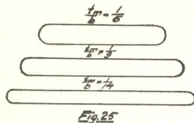
Sidoförhållanden. 1/6 är det sämsta användbara för Y = 15 \text{ dm}^2 och 1/14 det "bästa" användbara för stora modeller ( Y = 70 \text{ dm}^2 ).
