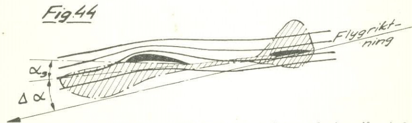
Planet intar därför detta läge i glidflykten, d. v. s. kropp och vinge får \Delta\alpha högre anfallsvinkel ( \Delta\alpha = nedsvepningsvinkeln).
