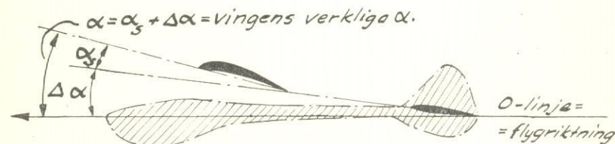
Vi sänker alltså redan på ritningen kroppens vinkel \Delta\alpha från den vinkel stabilisatorn avses flyga i, och beräknar anfallsvinkelskillnaden vinge—stabilisator ( \alpha_s ) så, att \alpha_s + \Delta\alpha blir den anfallsvinkel vingen bör ha i glidflykten.
