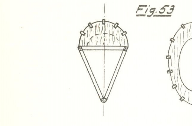
Fig. 53. Runda kroppssektioner. T. v. trekantig kropp med övre påbyggnad av halvcirkel-spant och formlistor. T. h. oval spantkropp i två halvor, vilka efter byggandet limmas ihop. Bägge kroppstyperna kan "plankas" med balsafanér.
