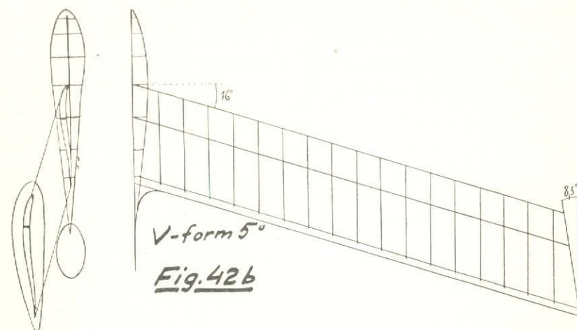
Fig. 42b Flygande vinge med utpräglad pilform, som bör kombineras med stark skränkning. Obs. vingprofilen, som genom sin uppböjda bakdel blir nästan tryckcentrumfast (och får sämre glidtal).
