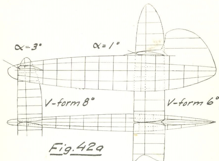
Fig. 42a S. k. anka, som flyger med höjdstyrverket först. Detta är bärande och har högre \alpha än vingen samt ett lägre \alpha_{max} . Modellens data är: b = 83 cm (vinge), 45 cm (stab.), L = 73 cm, G/Y = 16 g/dm 2 . Typen kräver en erfaren konstruktör.
