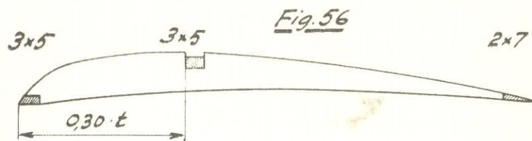
Profil: 6300B, t=140 mm, Sprygel av 0,8 mm asp.
