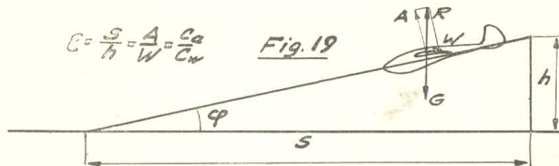
Ett flygplan glider sträckan s från höjden h . Genom triangelarnas likformighet blir förhållandet detsamma (lyftkraft/motståndet).
