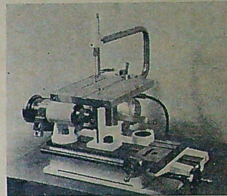
Maskinen med kontursågen monterad.
