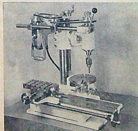
Pelarbormaskin med rundmatningsbord.
