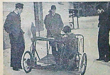
En bild från bilens byggnad, varav den enkla stålörskonstruktions klart framgår.
