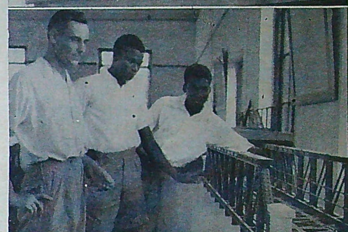
Brobyggnader spelar en stor roll i dessa delar av världen och för undervisningen på detta område håller man sig med en europeisk expert, mr Bickerstaff, som här demonstrerar en bromodell för ett par elever.
