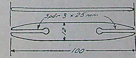
Fig. 10. Skytteln.
