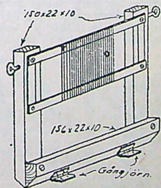
Fig. 8. Färdig vävsked.
