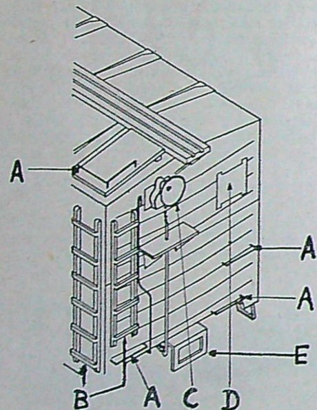
Fig. 1. Detaljer på godsvagn. A plattformshandtag av 0,2 mm metalltråd. B stegar. C bromsratt. D Vagnmärkestavla. E Koppelögla.
