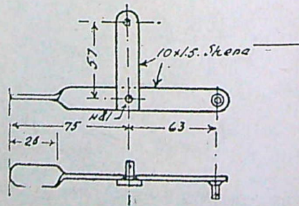
Fig. 6. Hävarmarna tillverkas av 10x1,5 mm mässingskenor.
