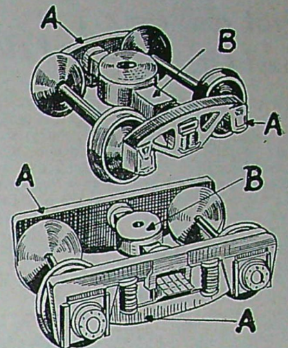
Fig. 8. Överst godsvagnsboggi, typ Bettendorff. Underst personvagnsboggi, 2-axlad. A bogglisidor. B mellanstycken.
