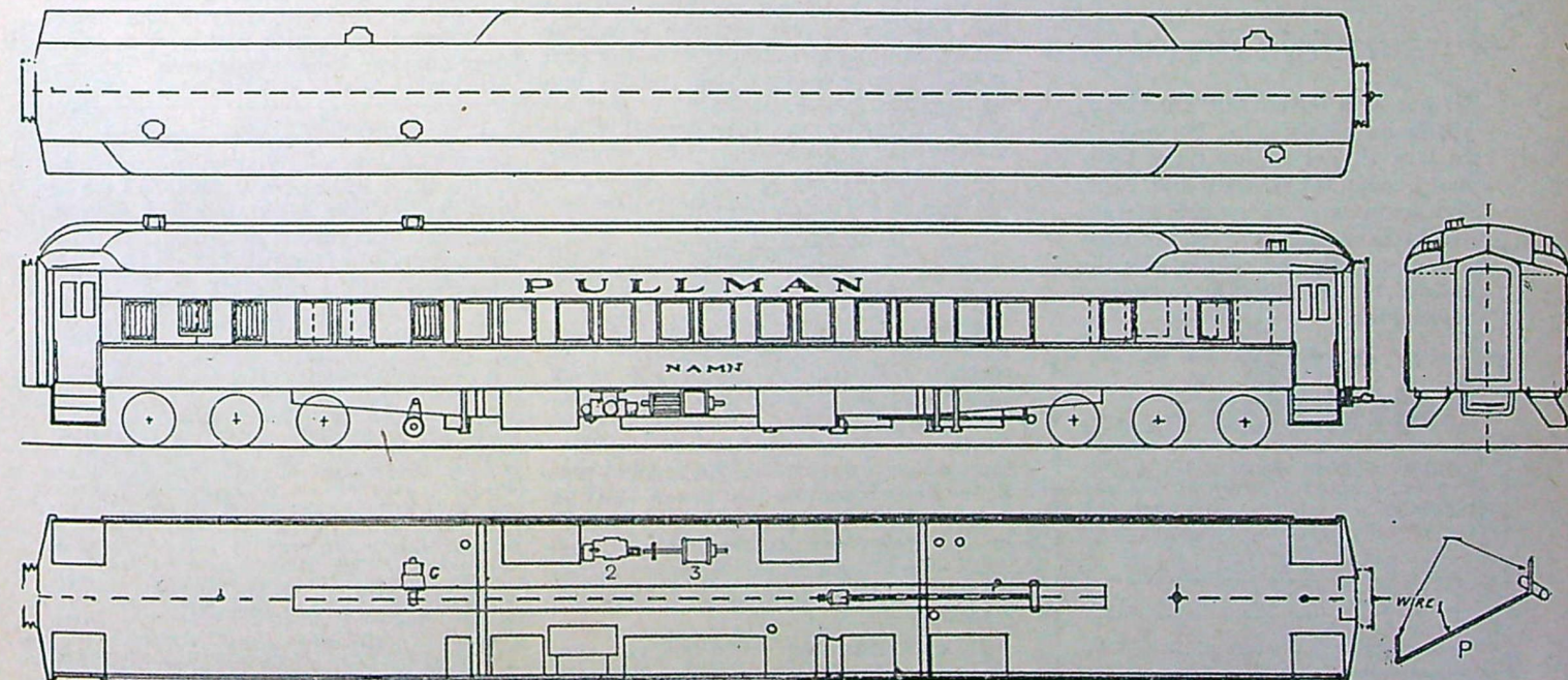
Fig. 9. Sammansättning av pullmanvagnen. G generator. 2 och 3 bromsdetaljer. P generatörledning.
