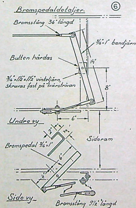
Sida vy - Bromspedal 3/16" långd
