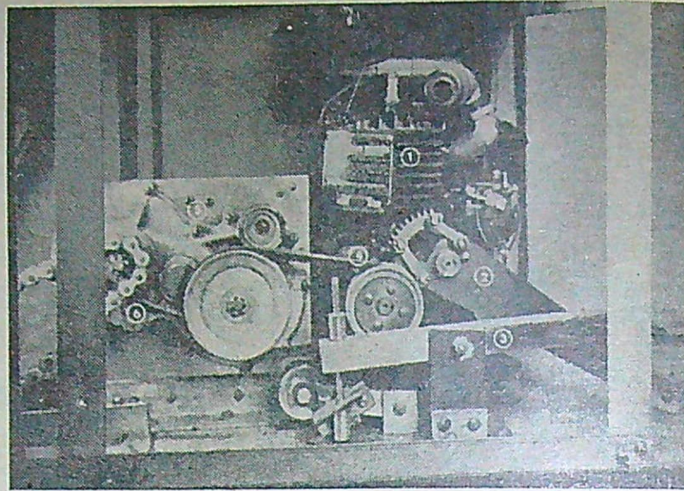
T. v.: Tryckfjädrar placeras mellan fjäderstödet och bakhjulsramen. T. h.: Det ena alternativet för maskinell utrustning. 1) Motor. 2) Kickstart. 3) Koppling. 4) Drivrem. 5) 1:1 Växellåda. 6) Kedja till drivhjulet. Det andra alternativet erhålls i ritning nr 8.
