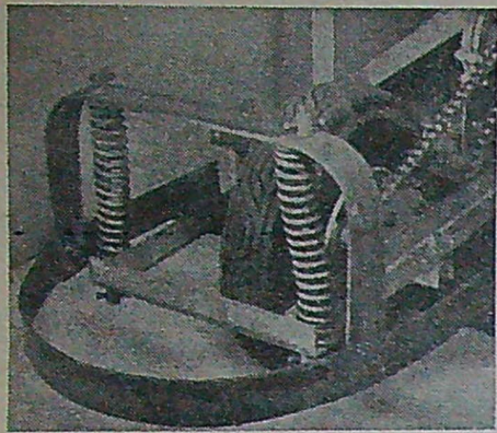
T. v.: Tryckfjädrar placeras mellan fjäderstödet och bakhjulsramen. T. h.: Det ena alternativet för maskinell utrustning. 1) Motor. 2) Kickstart. 3) Koppling. 4) Drivrem. 5) 1:1 Växellåda. 6) Kedja till drivhjulet. Det andra alternativet erhålls i ritning nr 8.
