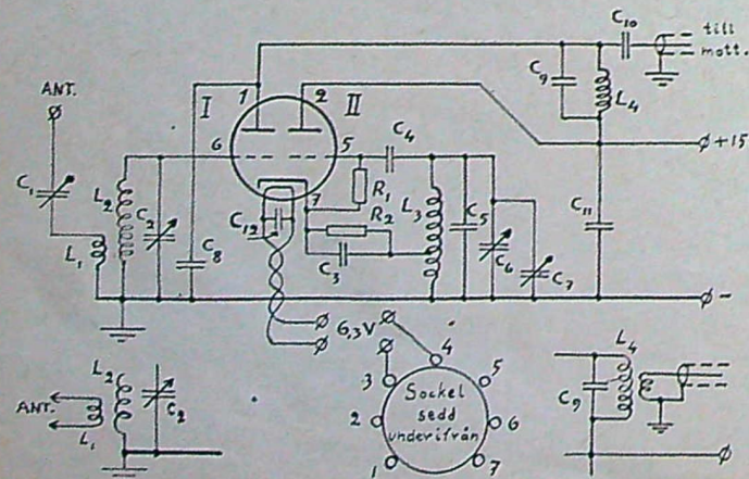
Fig. 1. C 1 =C 7 =30 pF trimmer C 2 =60 pF variabel C 3 =C 11 =0,05 µF C 4 =C 5 =50 pF glimmer C 6 =30 pF variabel C 8 =15 pF glimmer C 9 =storleksordn. 25 pF C 10 =30-50 pF C 12 =2 000 pF R 1 =50 kilohm ½W R 2 =500 ohm (ev. mind- re) ½W L 1 , L 2 , L 3 80 text. C 0 L 4 avstämmd till MF.
