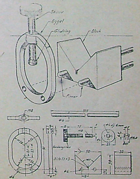
V-blocket färdigt för användning.
