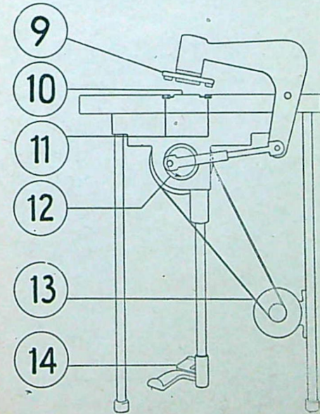
Schematiskt tvärsnitt av maskinen.
