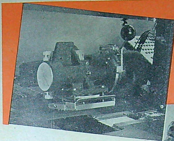
T. v.: Detaljbild av dubbelt tryckhuvud på en Citograf. Det ena tryckhuvudet är försett med en förnämlig nyhet — en radöverföringsanordning avsedd för arbetsplaneringssystem. Nedan en Citograf präglingsmaskin i vilken plåtarna präglas.
