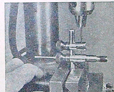
Montera benet och justeringsstödet på en 8 mm tapp när hålet för justerings-skraven ska borraras.
