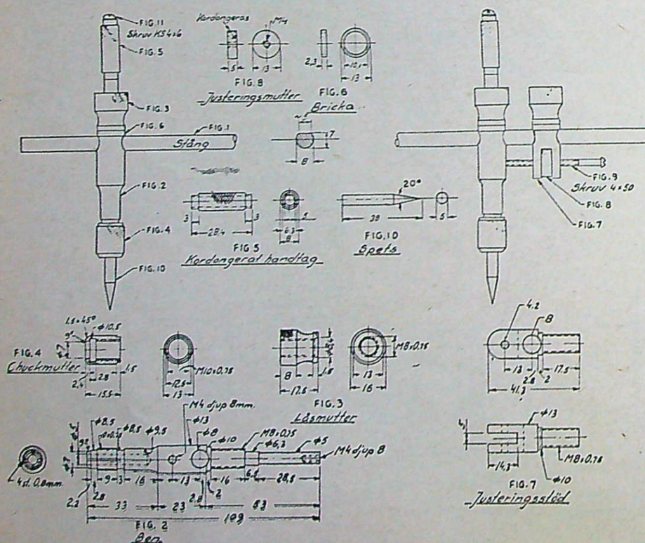
Svarva de två benen av 13 mm material, och använd en 13 mm spännpatron så som bilden visar eller en 3-backschuck under svarvningen och bearbetningen.
