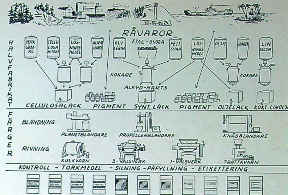
En schematisk framställning av färgtillverkningen.
