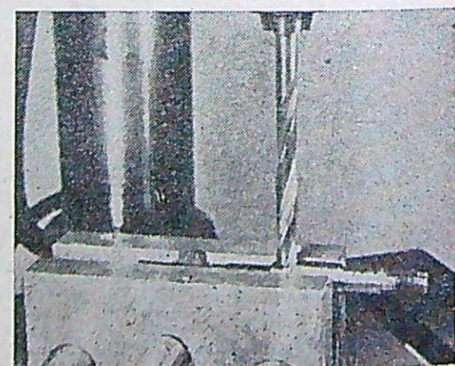
Vardera benet måste nu spännas in i ett borrarstykke när 8 mm hålet ska borraras och brotschas för glidpassning mot 8 mm stången.
