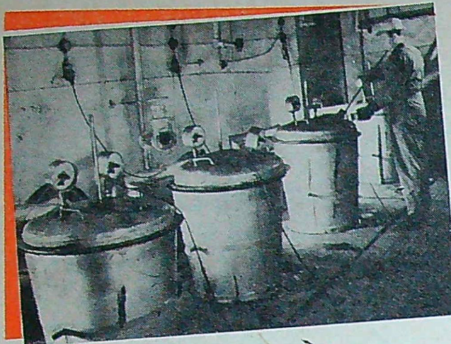
T. v. den s. k. "Smälten", där oljefärgen tillverkas. T. h. sker nyanseringen i cellulosalackfabriken.
