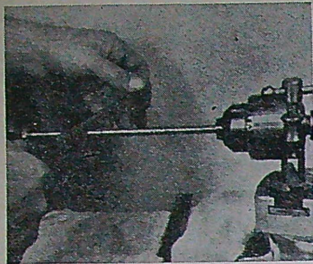
T. h. den färdiga stångcirkeln i användning. T. v. Spänn in 8x325 mm stången i svarven och fila 5 mm plana ytan. Kontrollera omsorgsfullt, om möjligt med mikrometer.
