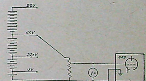
Fig. 5. Uppkopplingen vid kalibrering. Som spänningskälla används ett anodbatteri på 90 volt.
