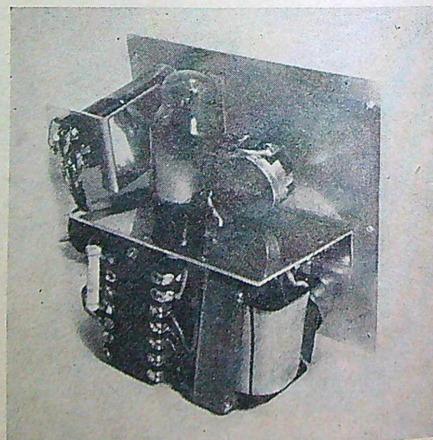
Fig. 3. Instrumentet utan låda, sett bakifrån. Överst till vänster ögat 6E5, monterat på en vinkel. Likriktarröret 6X5G är placerat stående.
