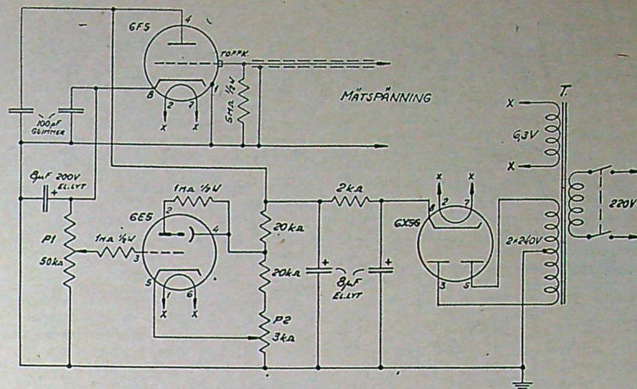
Fig. 2. Kopplingsschema. Vid likspänningsmätning ansluts plus till gallret på 6F5.
