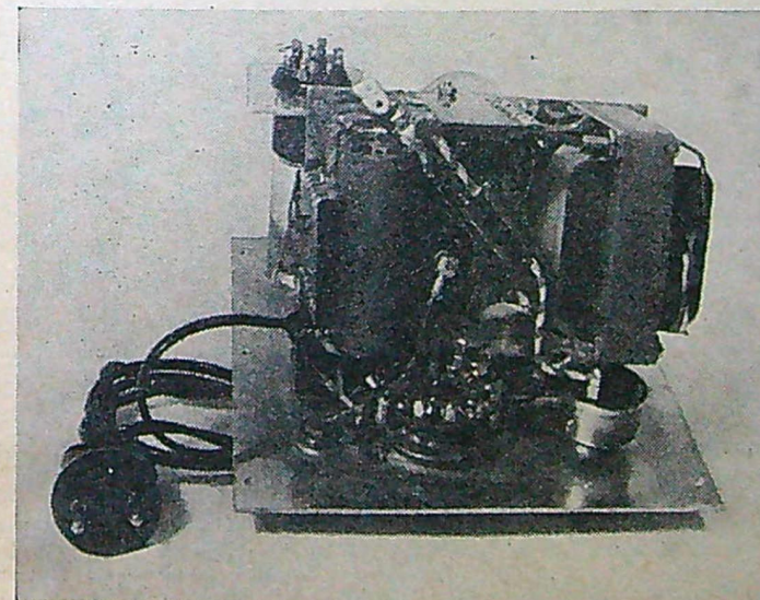
Fig. 4 (t. v.). Chassiet sett underifrån, nätaggregat, 6F5 och kopplingsplintar är hängande monterade.
