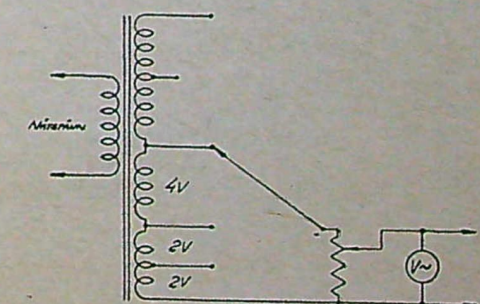
Fig. 6. Som spänningskälla för växelspannings skalan används en radiotransformator.
