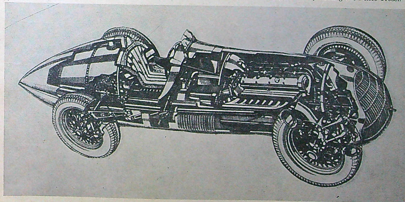
Röntgenbild av Alfa Romeos Typ 158 Alfette, efterkrigstidens snabbaste banracer i 1,5 liters-klassen.
