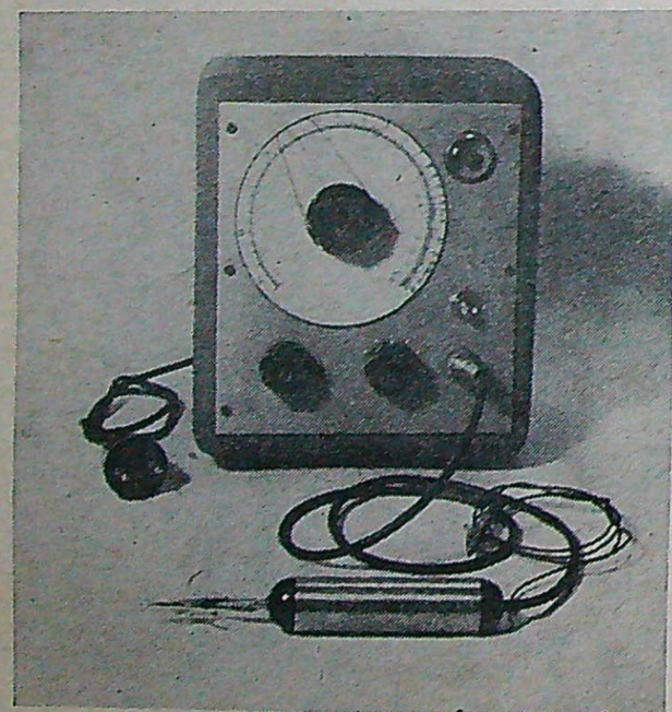
Fig. 1. Rörvoltmeters yttre. I mitten syns spännings skalan (P 1), under denna till vänster nolljusteringen (P 2) och till höger en omkopplare för en ev. spänningsdelare. Överst till höger syns ögat, där under nätströmbrytaren och mikrofonkontakten. Testkroppen på bilden används endast som "handtag".
