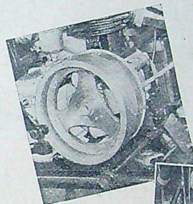
Ovan: Den påkrympta lättmetalltrumman åstadkommer en trumma, inuti vilken en friktionsback roterar vid starten och av centrifugalkraften slirar mot trummans vägg och sätter balanshjulet i rörelse.
