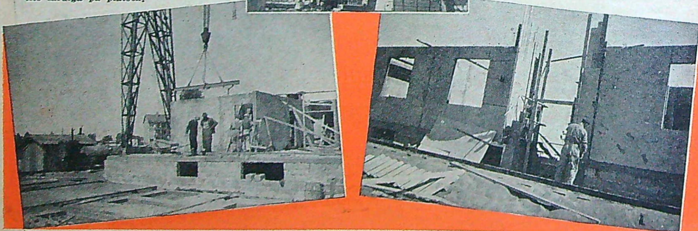
Bilden nedan visar sammanfogningen av de färdiggjorda väggsektionerna.
