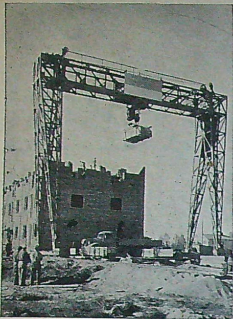
Ett med tegel fullastat bilflak går upp direkt till tredje våningen med bockkranens hjälp.
