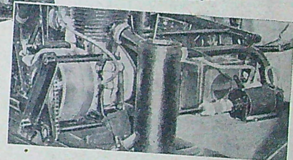
Ovan: Den påkrympta lättmetalltrumman åstadkommer en trumma, inuti vilken en friktionsback roterar vid starten och av centrifugalkraften slirar mot trummans vägg och sätter balanshjulet i rörelse.
