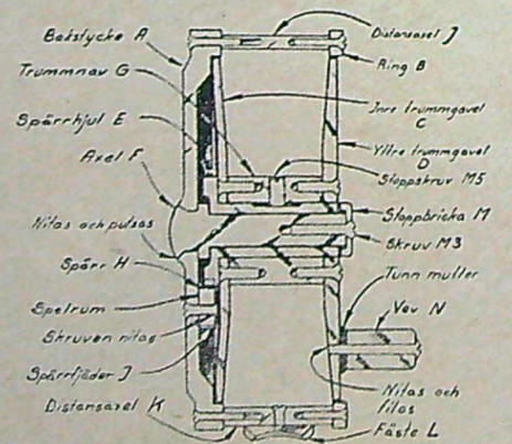
Sammanställningsritning för spinnrullen
