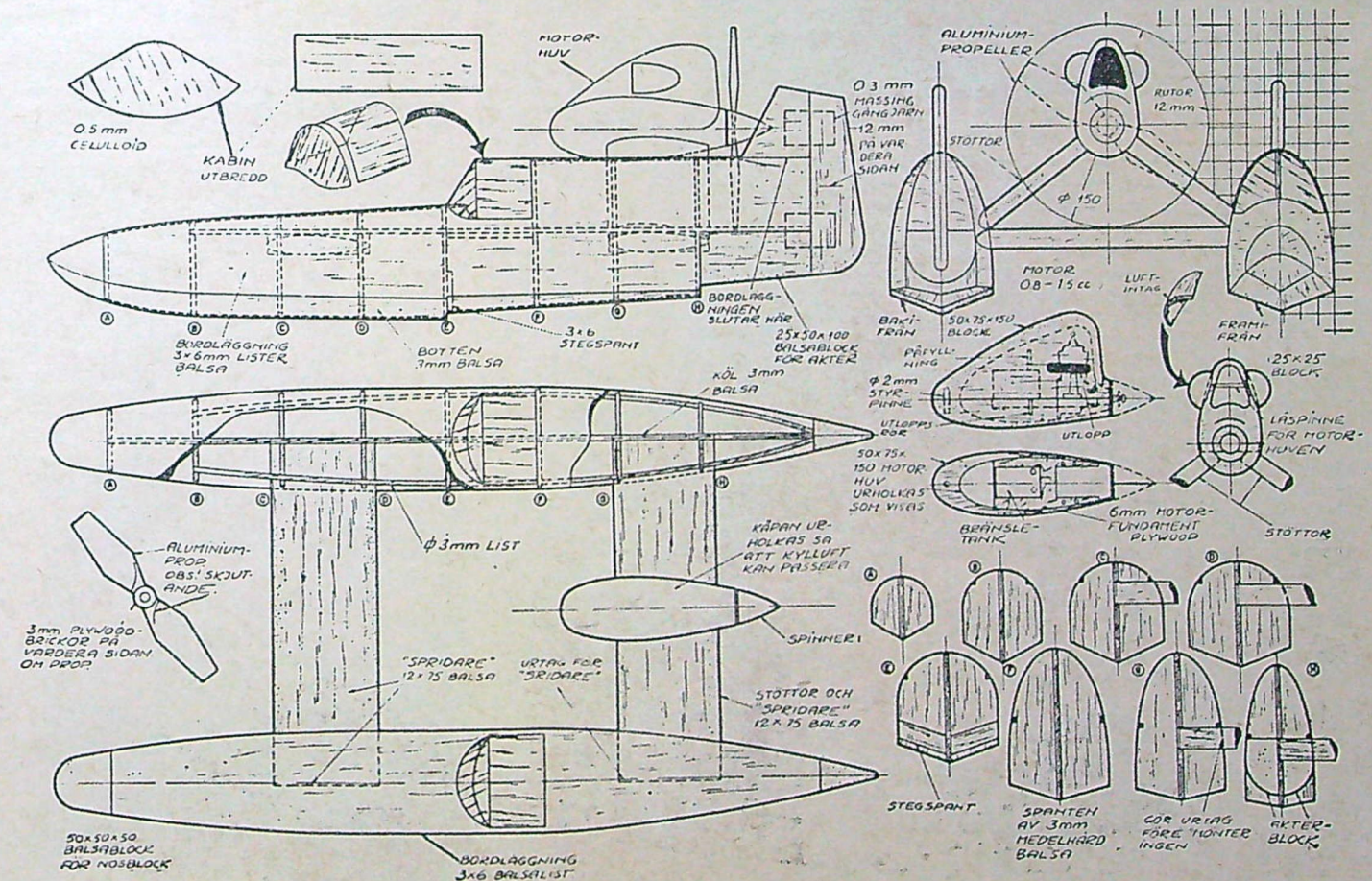
Översiktsritning av katamaranen.
