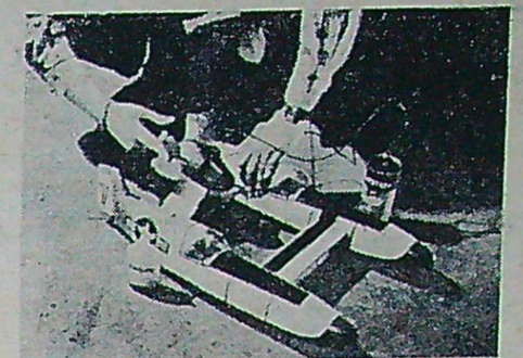
Fig. 4. Motorn kommer att starta mycket lätt genom att man ansluter ett vanligt batteri till glödpluggen och jord, om det nu är en diesel med glödplugg.
