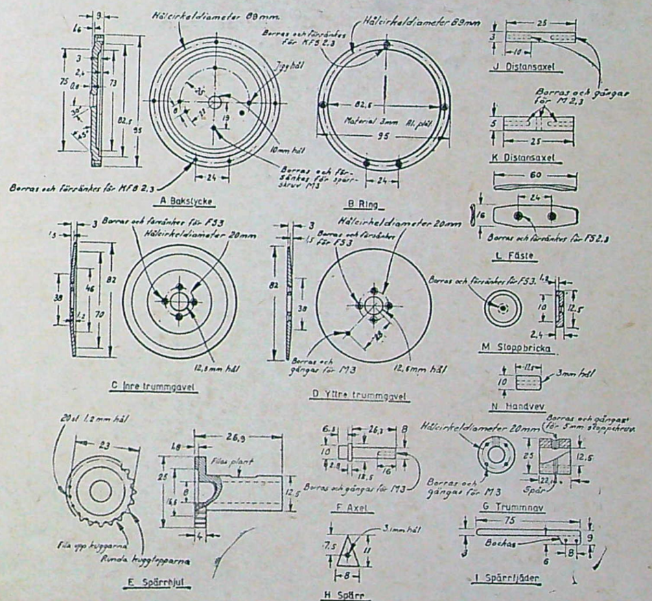
Måttsett ritning på spinnrullen.
