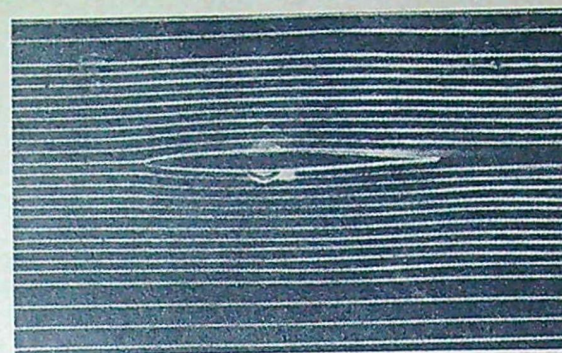
Fig. 2: Här visas en tunn vinge vid två olika anfallsvinklar. T. v. är vinkeln 0°, och t. h. är den 12°. Stall uppträder för tunna vingprofiler vid avsevärt lägre anfallsvinklar.
