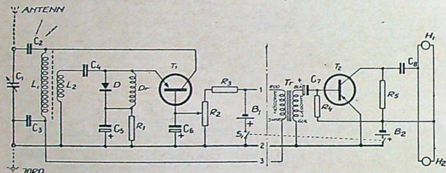
I fig. 1 t. v. ses kopplingsschemat för hatt-radion, medan fig. 2 nedan visar hur radions olika delar monteras på en efter hattens form böjlad tunn aluminiumplåt.
