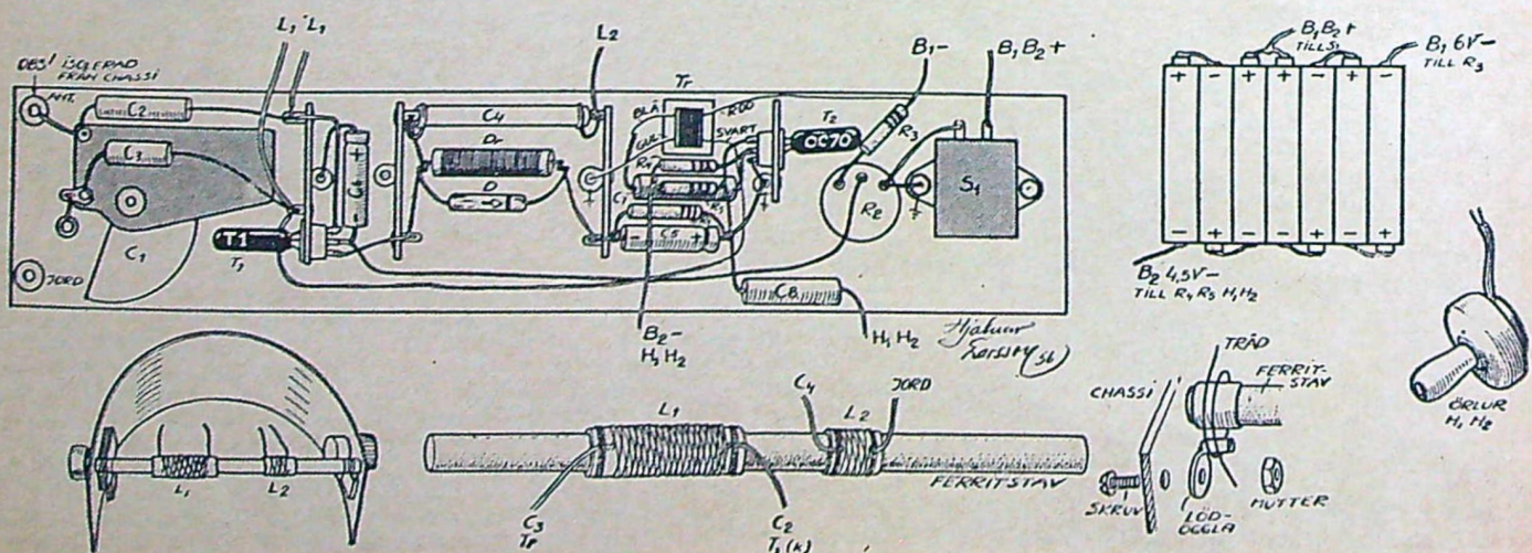
I fig. 1 t. v. ses kopplingsschemat för hatt-radion, medan fig. 2 nedan visar hur radions olika delar monteras på en efter hattens form böjlad tunn aluminiumplåt.
