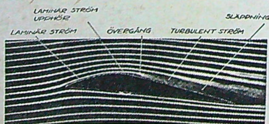
Fig. 3 (t. v.): Detta fotografi visar, hur gränsskiktet på profilens översida plösslut gör strömningen turbulent.
