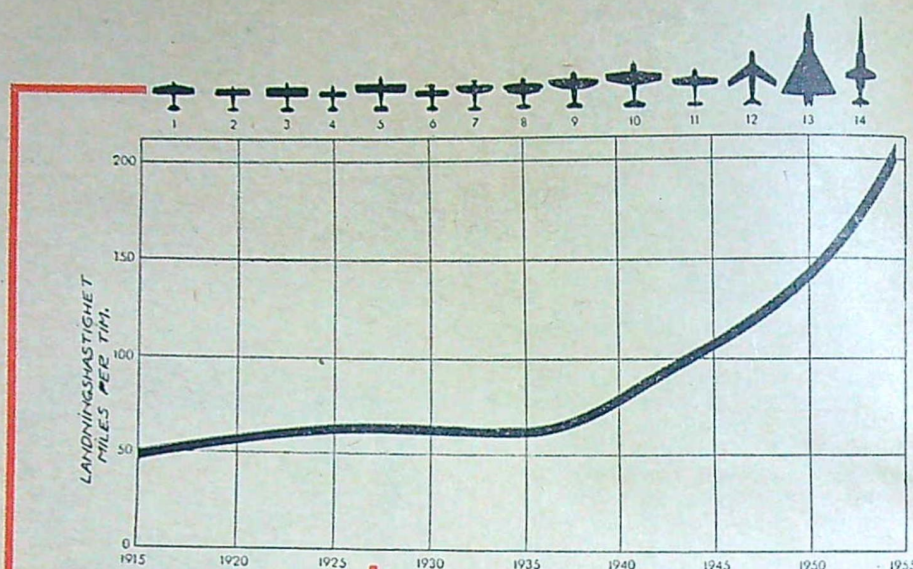
Fig. 8 (ovan): Landningshastigheten har stigit kraftigt från 1915. Varje silhuetbild visar kända flygplan rakt över deras landningshastigheter. Från vänster följande flygplan: 1) S.P.A.D. 2) Thomas Morse MB-3. 3) Curtiss Pursuit. 4) Curtiss R-2C-1 Navy Racer. 5) Charles Lindberghs Spirit of St. Louis. 6) Geo Bee Senior Sportser. 7) Boeing P-26. 8) Curtiss Hawk Type IV. 9) Seversky 2 P.A.-L. 10) Grumman Hellcat. 11) Focke-Wulff 190. 12) F-86. 13) F-102. 14) Douglas X-3.
