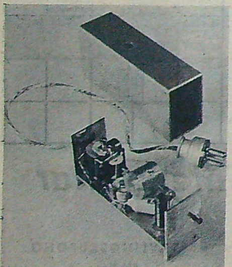
Mottagare för radiostyrning av modeller.
