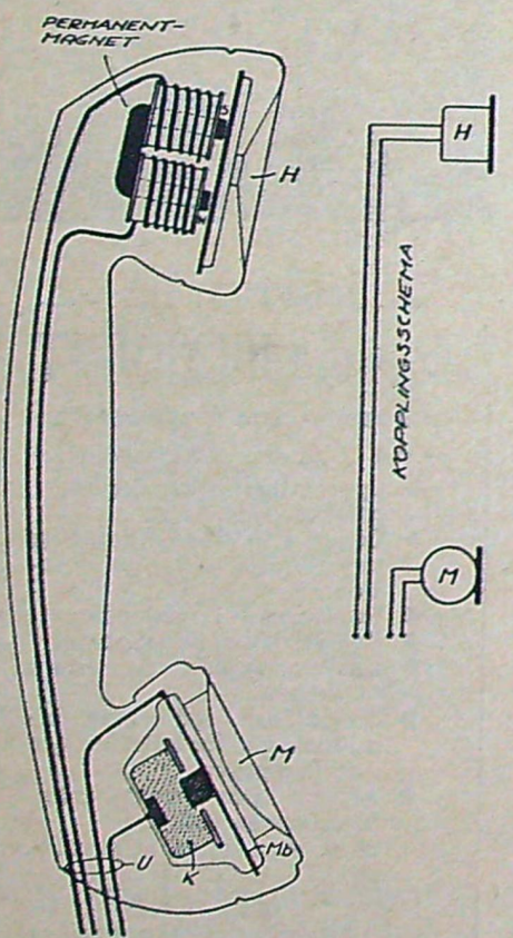
Fig. 1. Genomsnitt av mikrotelefon.
