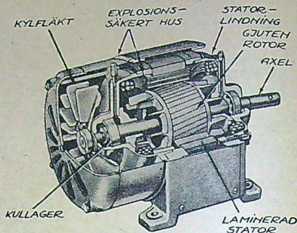
En enfas asynkronmotor med induktiv startlindning.
