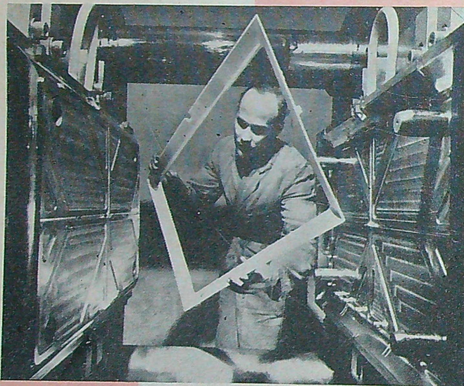
En färdigsprutad kylskåpsram av termoplast lyfts just ut ur den öppnade formen vid Skånska Åttikfabriken i Perstorp.
