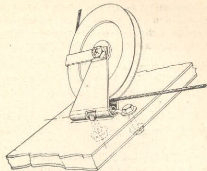
Fig. 6. Bryttrissa för styrlina.
