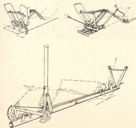
Fig. 4 och 5. Sidoroderpedalerna i olika utföranden. Handspaken.
