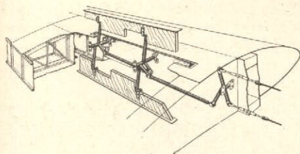
Fig. 2. Bromsklaffarnas konstruktion.
