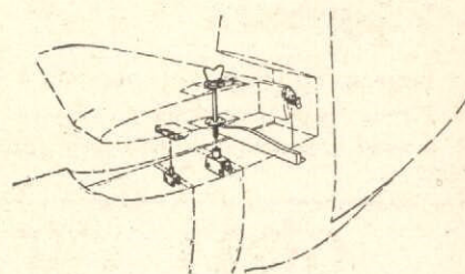
Fig. 8. Stabilisatorns montering vid kroppen.
