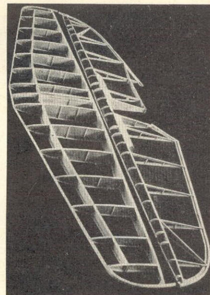
Fig. 7. Stabilisator och höjdroder utan klädsel.
