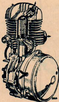
Ovan: Genomskärning av tyska Triumph-motorn som visar Ingasportarna och spolsystemet. — T. h. tvåtaktsprincip använd bl. a. av Puch. — Nedan en genomskärning av DKW:s kanske populäraste maskin, NZ 350, från år 1938.
