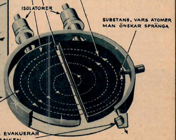
SCHEMATISK TECKNING AV VAKUUMKAMMAREN (placerad mellan polerna av en elektromagnet)
