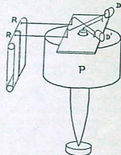
Schematisk bild av Wiechert-seismografen, där P är pendeln (1 600 kg), D dämpningskolkvar och R ritstift.
