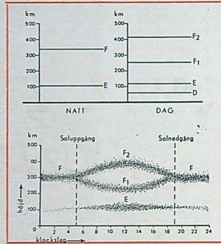
Ovan: Diagram, utvisande skikthöjderna i jonsfären. Som synes är variationerna mellan dag och natt mycket stora, och övergången är starkt markerad vid solens uppgång och nedgång.
