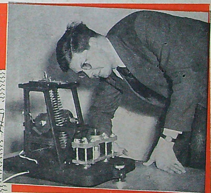
Nedan docent Marcus Båth vid Uppsalainstitutionens elektromagnetiska gretenseismograf, med instrumentets skyddskåpa borttagen.
