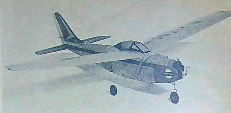
Completa är en nyhet från Hegl. Modellen är utförd i styroporskomplast med hårdträförstärkningar. Spännvidden är 95 cm och motorbockarna avpassade för 0,8 cc-motorn Piccolo. Lämplig radio är Metz Baby. Beckman & Co. 112:—.
