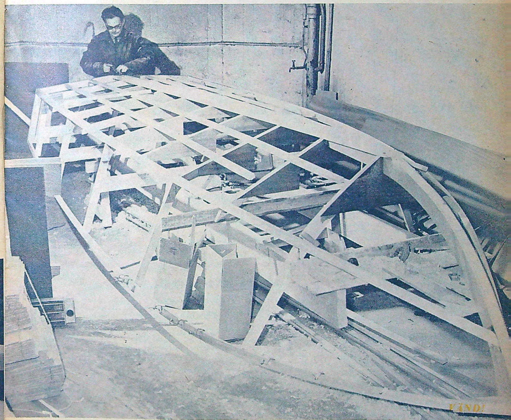
8 "Skelettet" till Alnö är färdigt. Plywoodbordläggningens anliggningsytor mot vägarna har snedhyllats och är nu i stort sett färdigjusterade. En bra hyvel med vasst skär rekommenderas när det gäller grovhyllningen av innerkölens, ett arbete, som bäst utförs sittande på kölen. För finjusteringen har man god användning av en rejäl rasp och en Surform-hyvel. Var noga med att kontrollera att skruvarna är ordentligt försänkta så att hyveln inte skadas.
