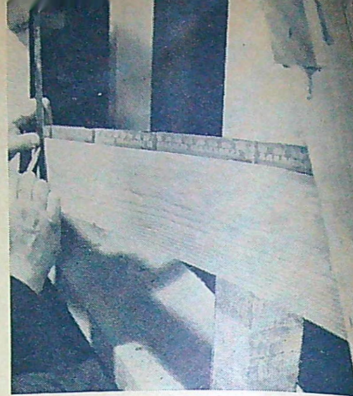
2 Mittpunkten på spantens bärplanka mäts upp. Använd vinkelhake och kontrollmät noga så att spantet blir rätt centrerat.
