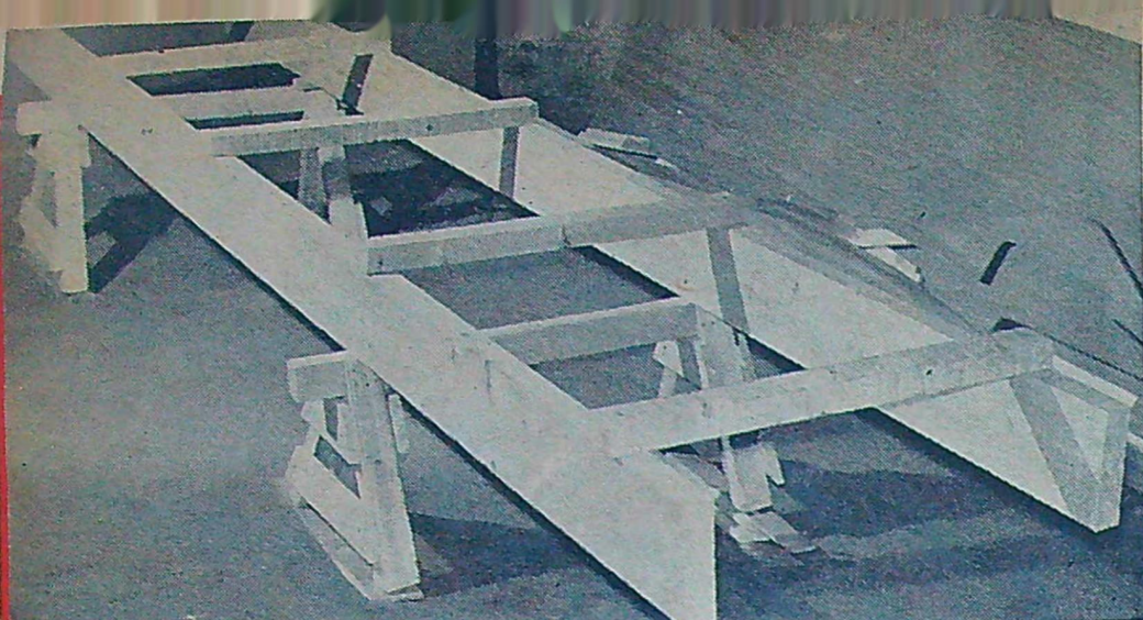
1 Arbetet inleds med tillverkningen av jiggen. Det är en byggstege som utförts av rejält tilltagna regler med "stegpinnar" av läkt. Den vilar på ett par robusta bockar och det är mycket viktigt att hela byggjiggen är fullkomligt horisontell. Det gäller här att grundligt använda vattenpasset.
