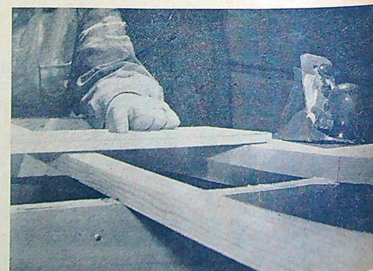
7 Slagvägare, innerköl och stäv måste snedhyllas så att plywoodborden ligger jämnt emot. Inturningen, dvs i det här fallet uppmätningen av snedhyllningsgraden, sker genom att föra en list längs bottenvägarna.
