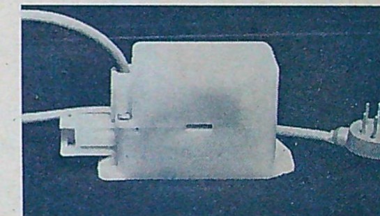
Metz Mecatron finns också i tre- och tiokanalssystem. Mecatron 195/3 är en helt ny servo för dessa flerkanalssystem. Måtten är 2x3,6x5,6 cm och vikten är 60 g. Denna snabba 3-10-kanalsservo kostar 56 kronor. B Beckman & Co AB.
