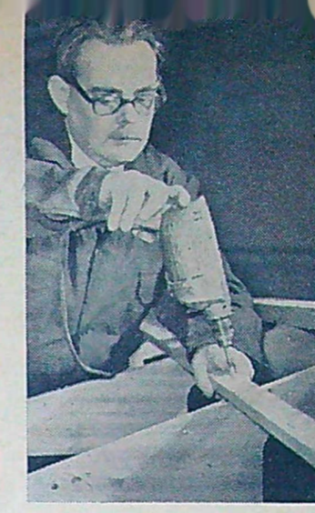
4 Efter det att innerkölens lagts på skruvas och limmas fyra bottenvägare mot spanten.
