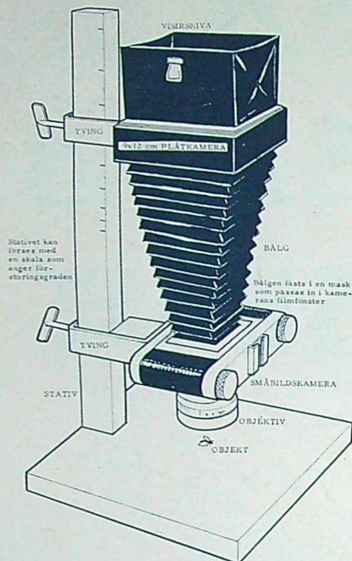
Mikrokameran består av en 9x12 cm plåtkamera med bälge, en småbildskamera samt ett trästativ. Kameran ger mikrobilder av mycket hög kvalitet.
