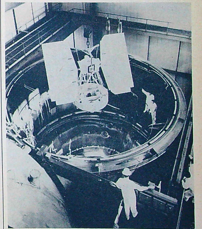
På flygutställningen i Paris demonstrerades denna modell i full skala av vädersatellit Nimbus, som på bilden sänks ner i världens största rymdsimulator. Denna är konstruerad av General Electric i USA och gör det möjligt att efterlikna de förhållanden som råder i rymden med avseende på vakuump, temperatur och solstrålning. Genom att sänka ner en satellit eller rymdfarkost i simulatortorn kan man se exakt vad som kommer att hända den när den kommer ut i rymden.
