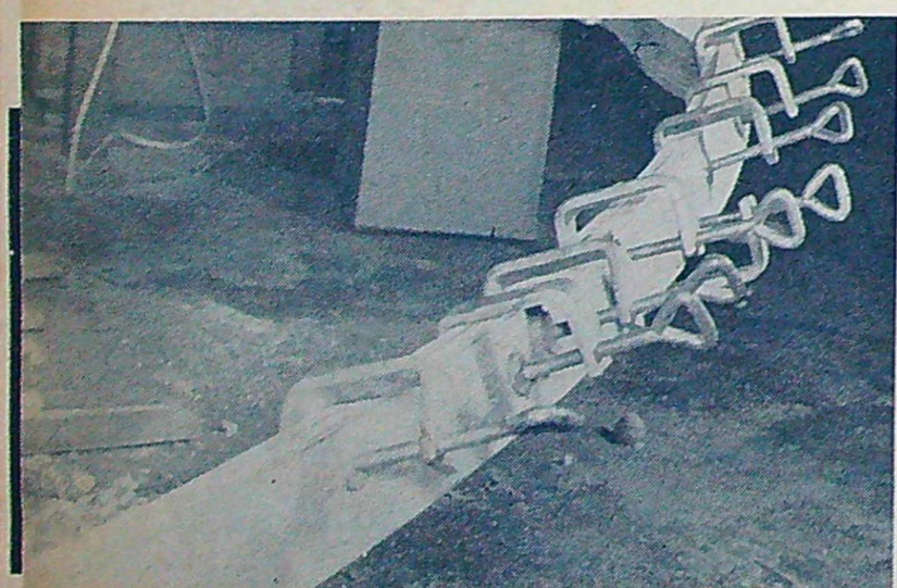
6 Balkvägaren (relingsinnerlisten) är kraftigt böjd in mot fören. För att underlätta arbetet är den utförd i två plywoodremmar, som limmas ihop. Här hålls listen samman med tvingar under det att limmet torkar.
