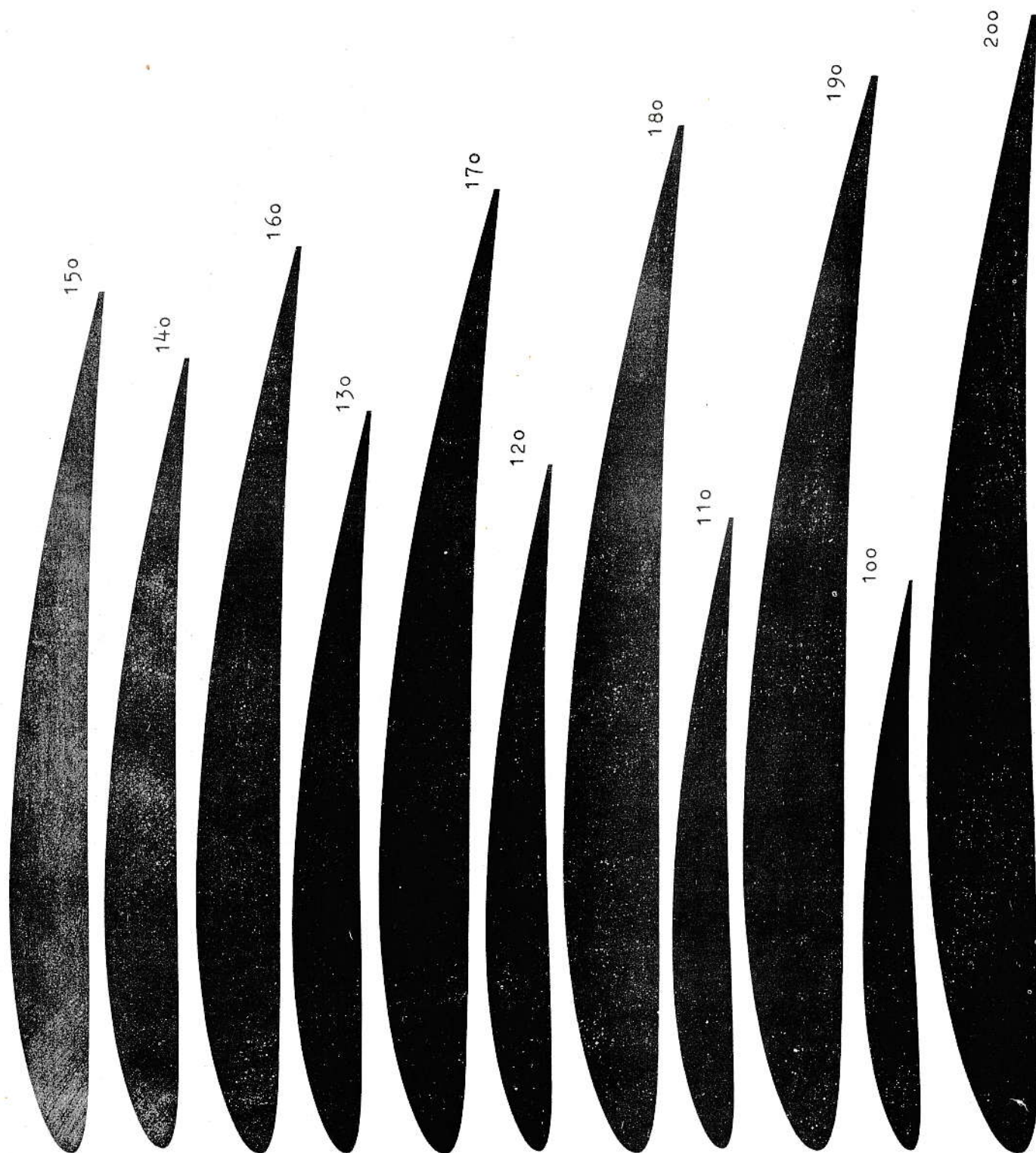
Profil N.A.C.A. 4409
